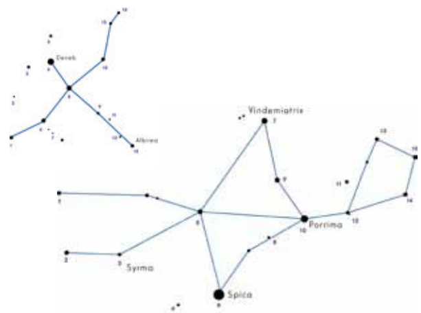
Constellation du Lion, du Cygne et de la Vierge © AFA | M.Evanno
